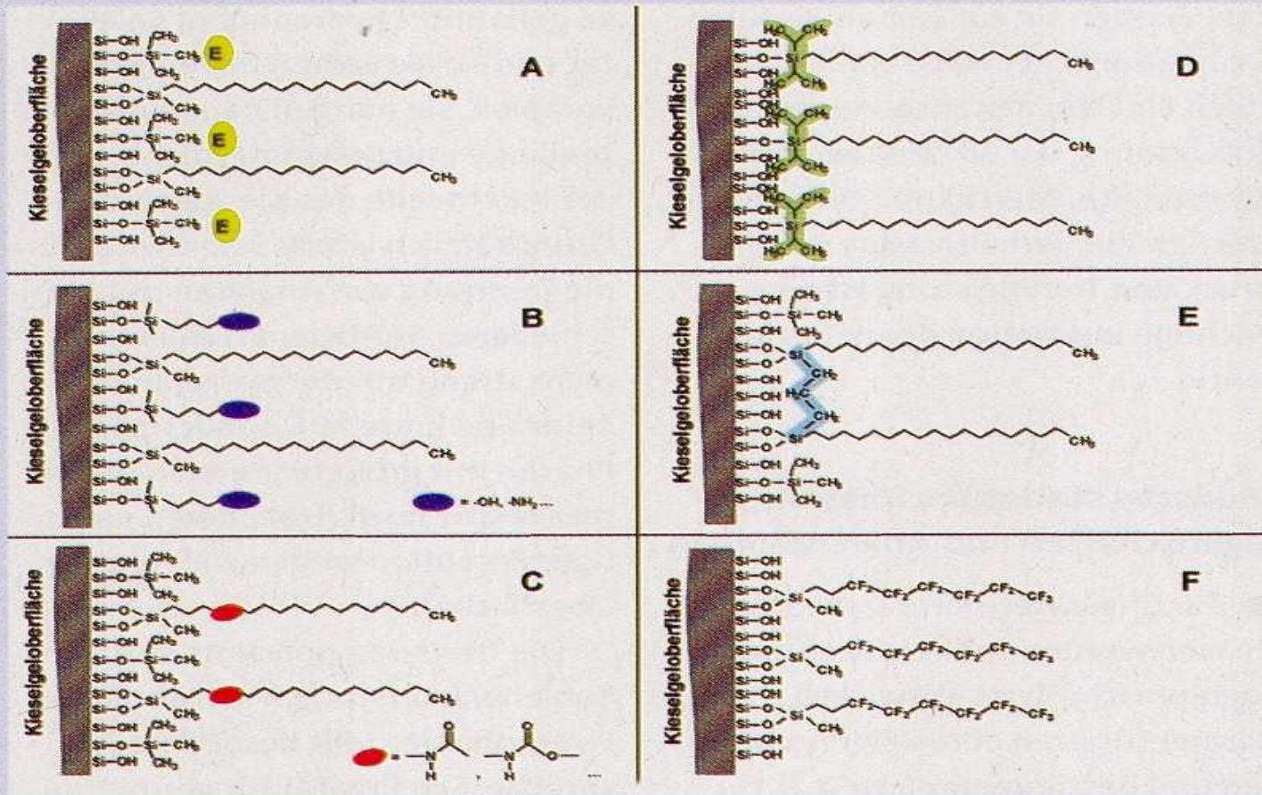
Abb. 1. Schematische Darstellung der Oberflächenmodifizierungen verschiedener Umkehrphasen: A) C18-Phase mit normalem Endcapping (E); B) C18-Phase mit hydrophilem Endcapping; C) C18-Phase mit eingebundenen polaren Gruppen („Shield Phase“); D) C18-Phase mit sterisch anspruchsvollen Seitengruppen („Bulky Groups“); E) Bidental verknüpfte C18-Phase; F) Fluoralkyl-Umkehrphase (C8).
